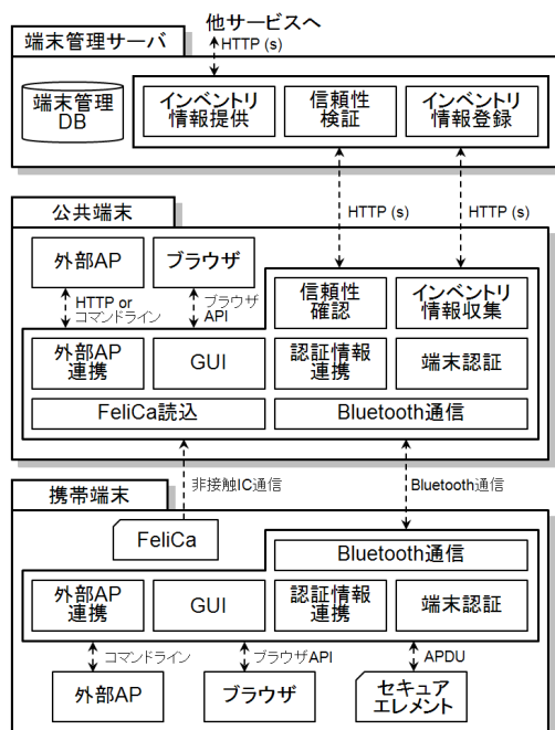
図 13 提案方式のモジュール構成
