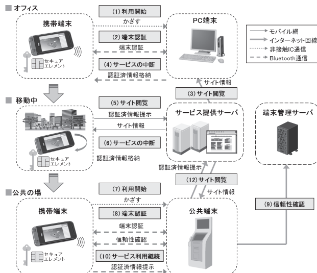
図 6 提案システムの全体概要 Fig. 6 Summary of proposed system.
